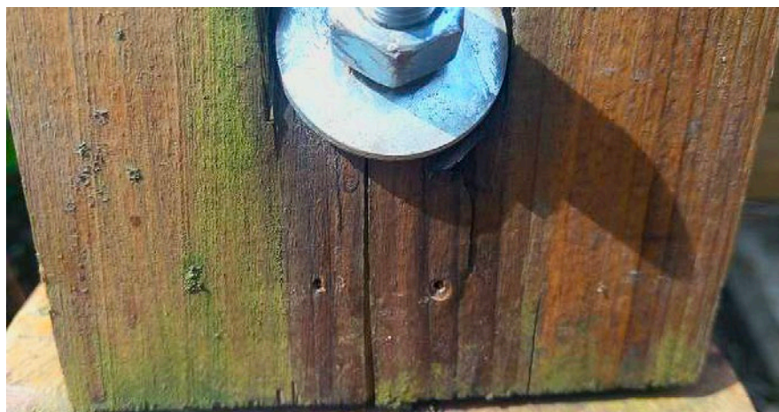
Příklad degradace konstrukčního dřeva hnědou hnilobou způsobená dřevokaznou houbou
