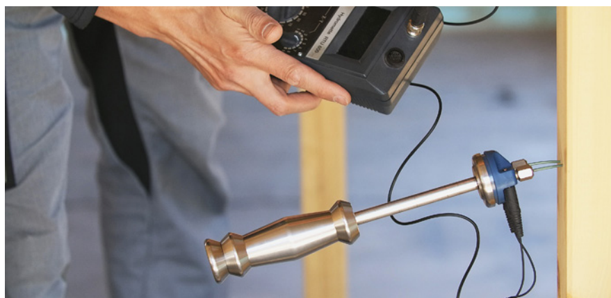
Vlhkost se může měřit i v konstrukci pro detekci nevhodně provedených konstrukčních detailů.
